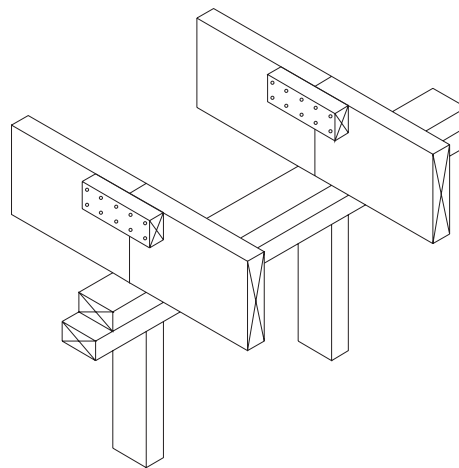
UNION DE VIGUETAS A TESTAS
