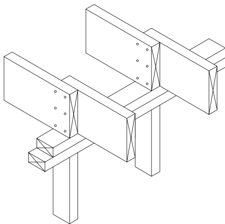
UNION DE VIGUETAS TRASLAPADAS
