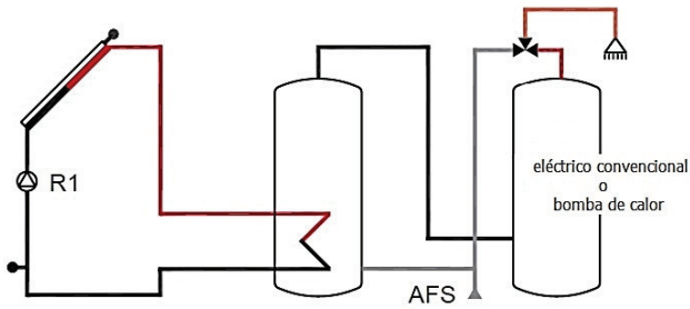
Sistema Solar con apoyo Eléctrico
