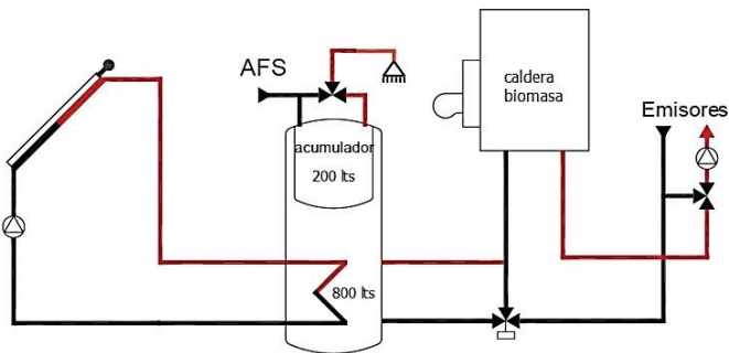
Sistema Solar ACS y Calefacción
